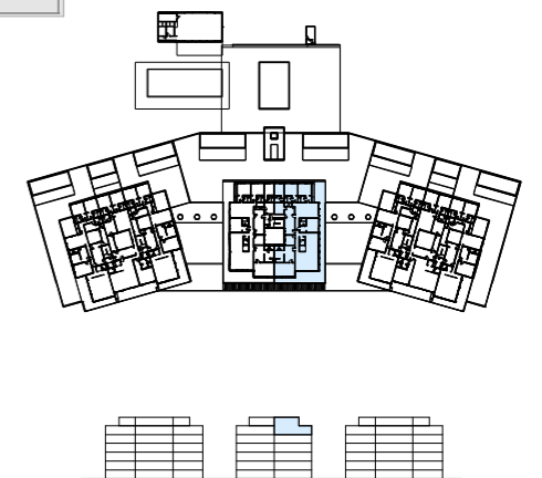
BLOQUEB - APTO. B602 + GÁLIBO
